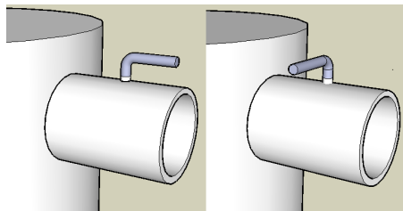
Otevřená poloha Uzavřená poloha Polohy ovládací páky pro nastavení hradítka (škrtecí klapky spalin) v kovuodu
