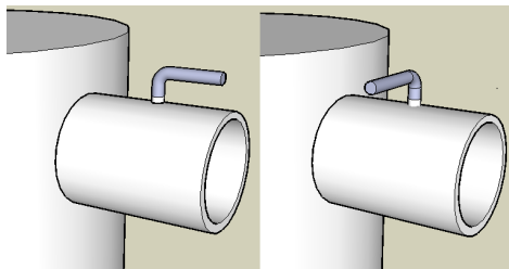
Avatud positsioon Suletud positsioon Siiber (heitgaaside piirdeklapi) reguleerimise kangi asendid lõõris
