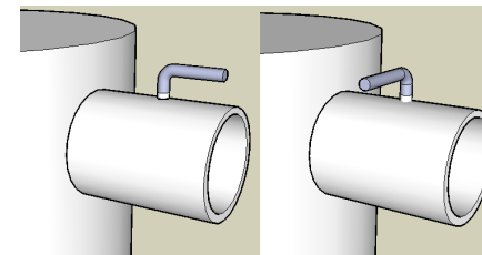
Atvērta pozīcija Slēgta pozīcija Aizbīdņa (dūmu droseles) regulēšanas roktura pozīcijas dūmvadā
